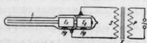
冷却水銀燈の發光管
